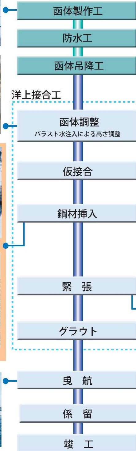
上床版鋼材挿入
