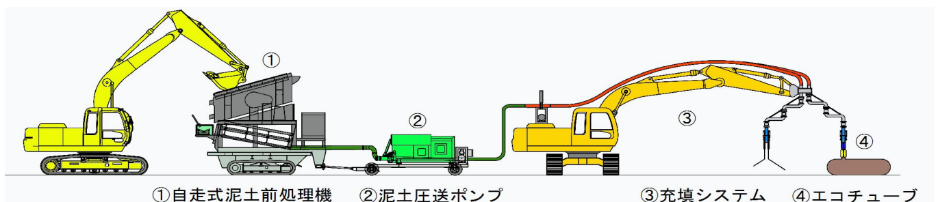
図-1 SPAD システム概要図
