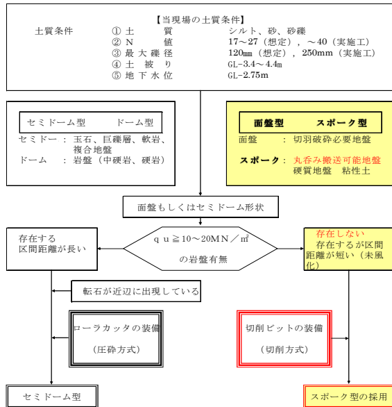
図-3 面盤形状の選定フロー
