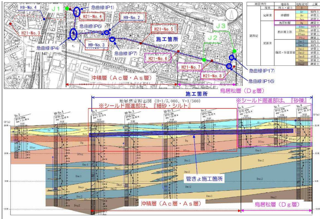
図-2 地層想定断面図
