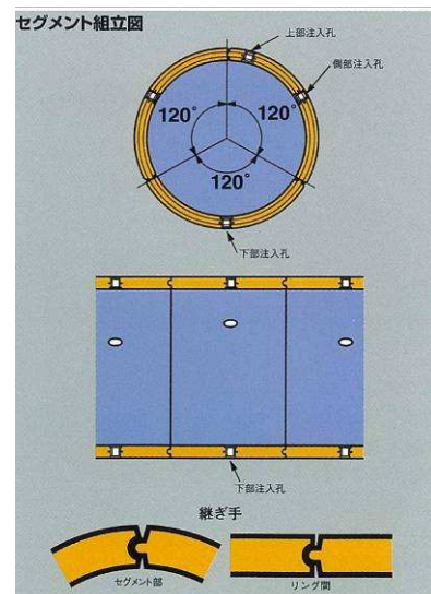
図-6 セグメント組立図
