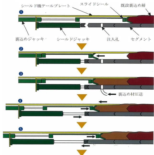
図-7 裏込め注入フロー図
