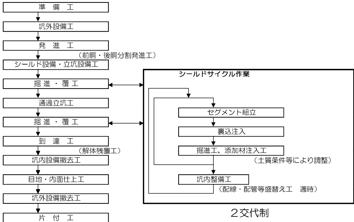
図-4 ミニシールド工法施工サイクル
