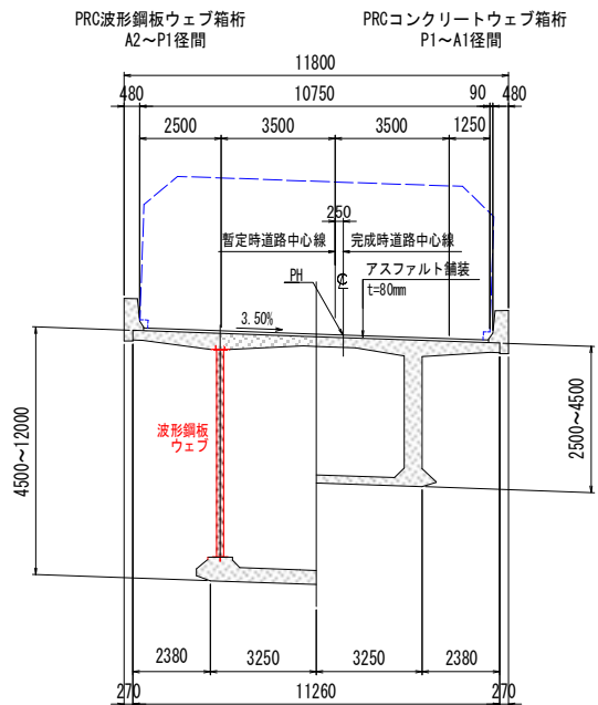
図-4 標準断面図
