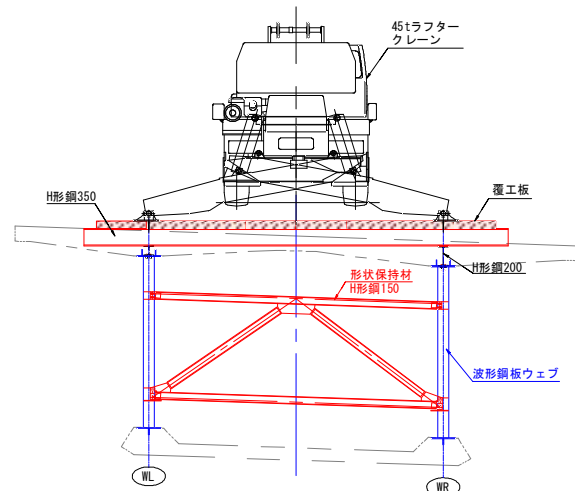
図-8 波形鋼板ウェブ上の作業概要図
