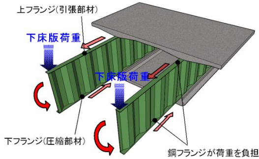
図-5 波形鋼板ウェブの耐荷機構
