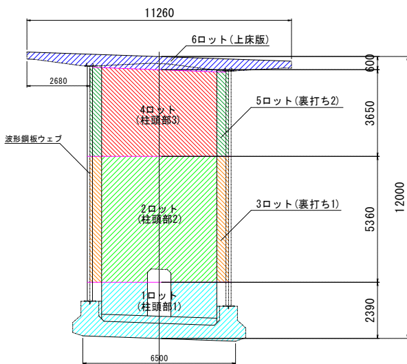
図-7 P2 柱頭部の分割施工概要図
