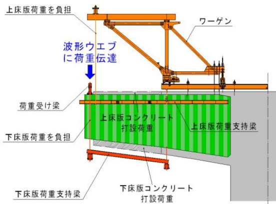
図-6 下床版コンクリートの支持構造
