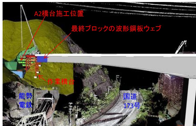
図-9 構台からの A2 施工状況概要図
