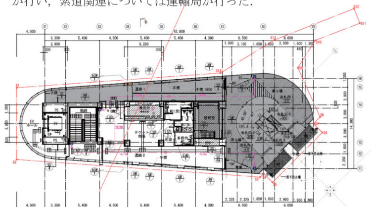
※塗りつぶした範囲は建築基準法適応外 （改札内，運転監視室及び格納庫他）
