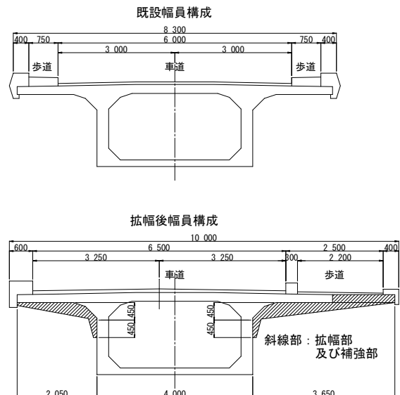
図-2 拡幅要領図
