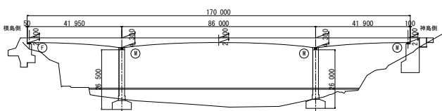
図-1 橋梁概要図
