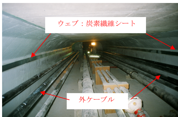
写真-2 主桁補強状況
