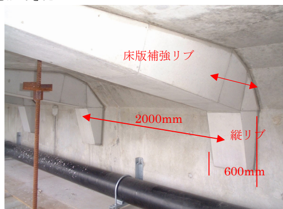
写真-3 補強リブ形状
