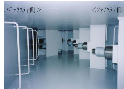
主塔鋼殻内の斜材定着体
