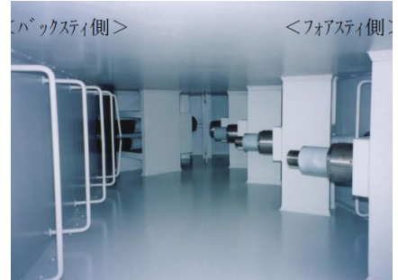
主塔鋼殻内の斜材定着体
